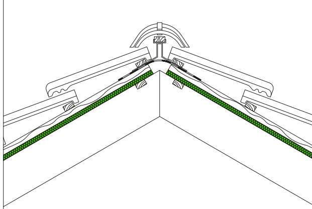
Panneau de sous-toiture STEICO
