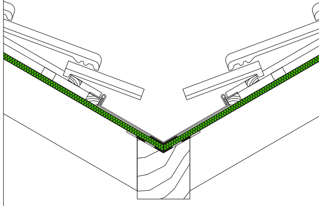
Panneau de sous-toiture STEICO
