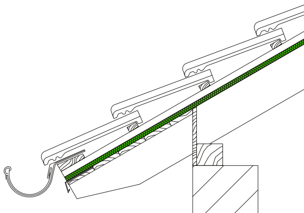
Panneau de sous-toiture STEICO
