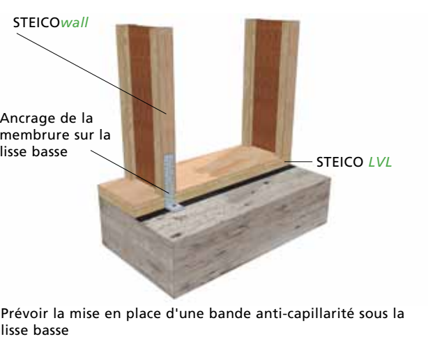
W4 Jonction sur dalle béton
